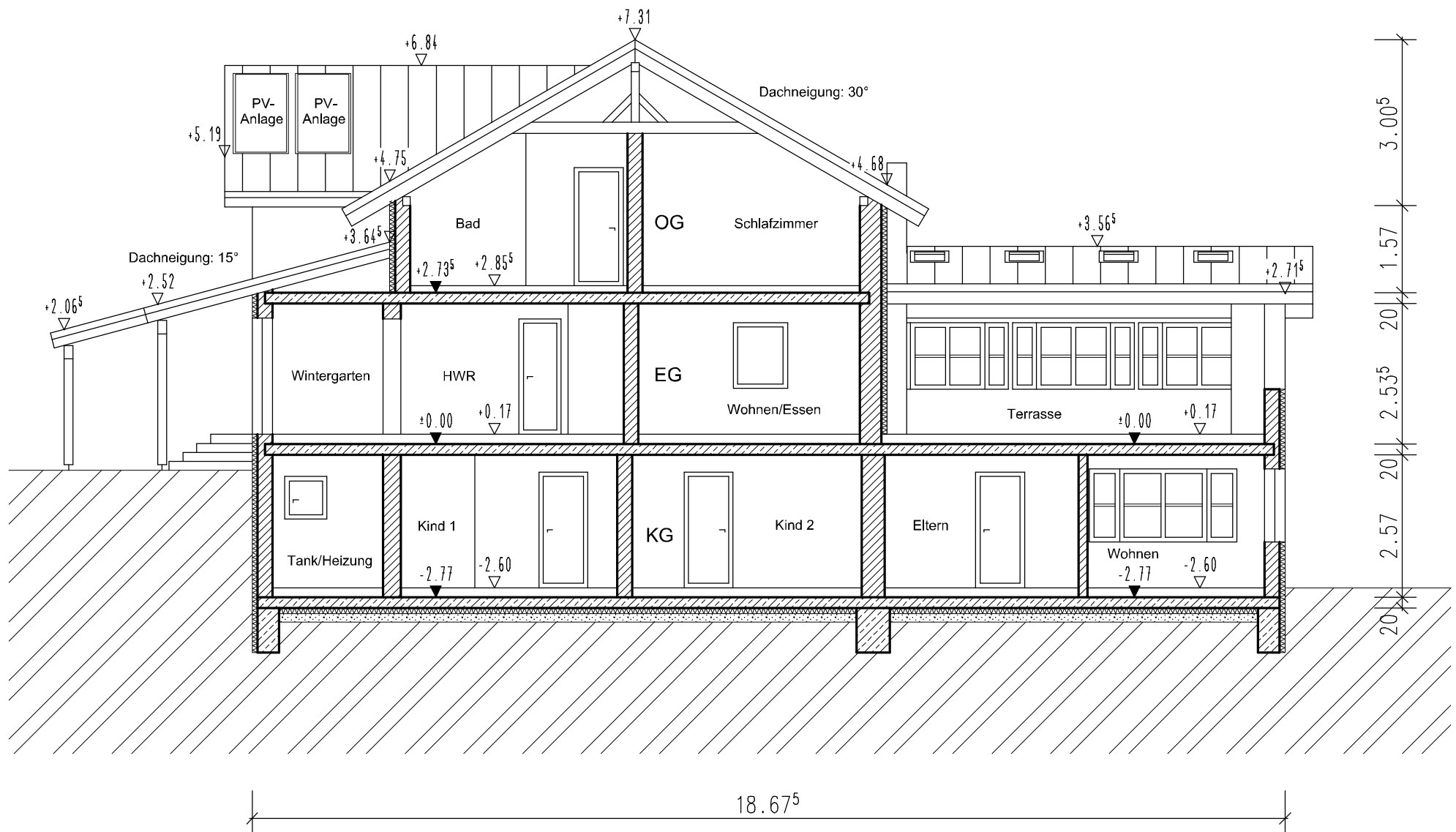
Schnitt A-A
