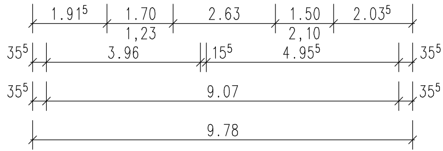
Grundriss UG
