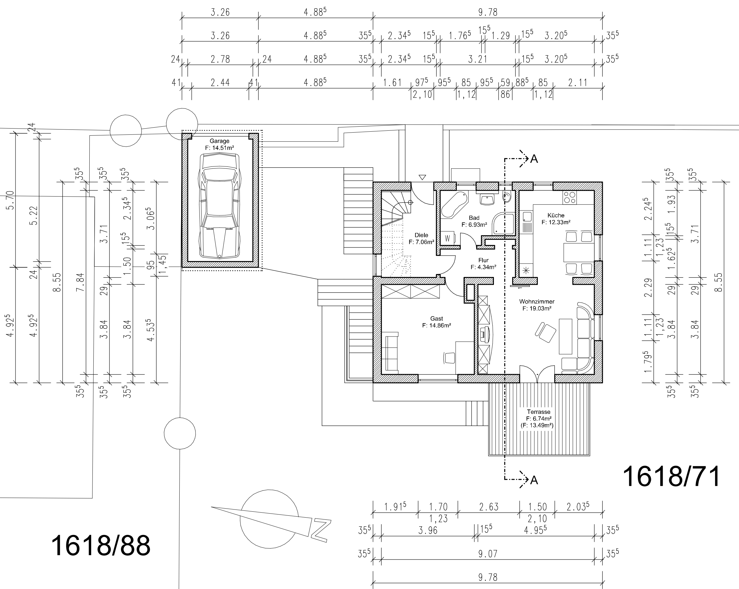
Grundriss EG
