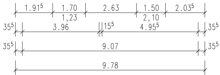
Grundriss EG
