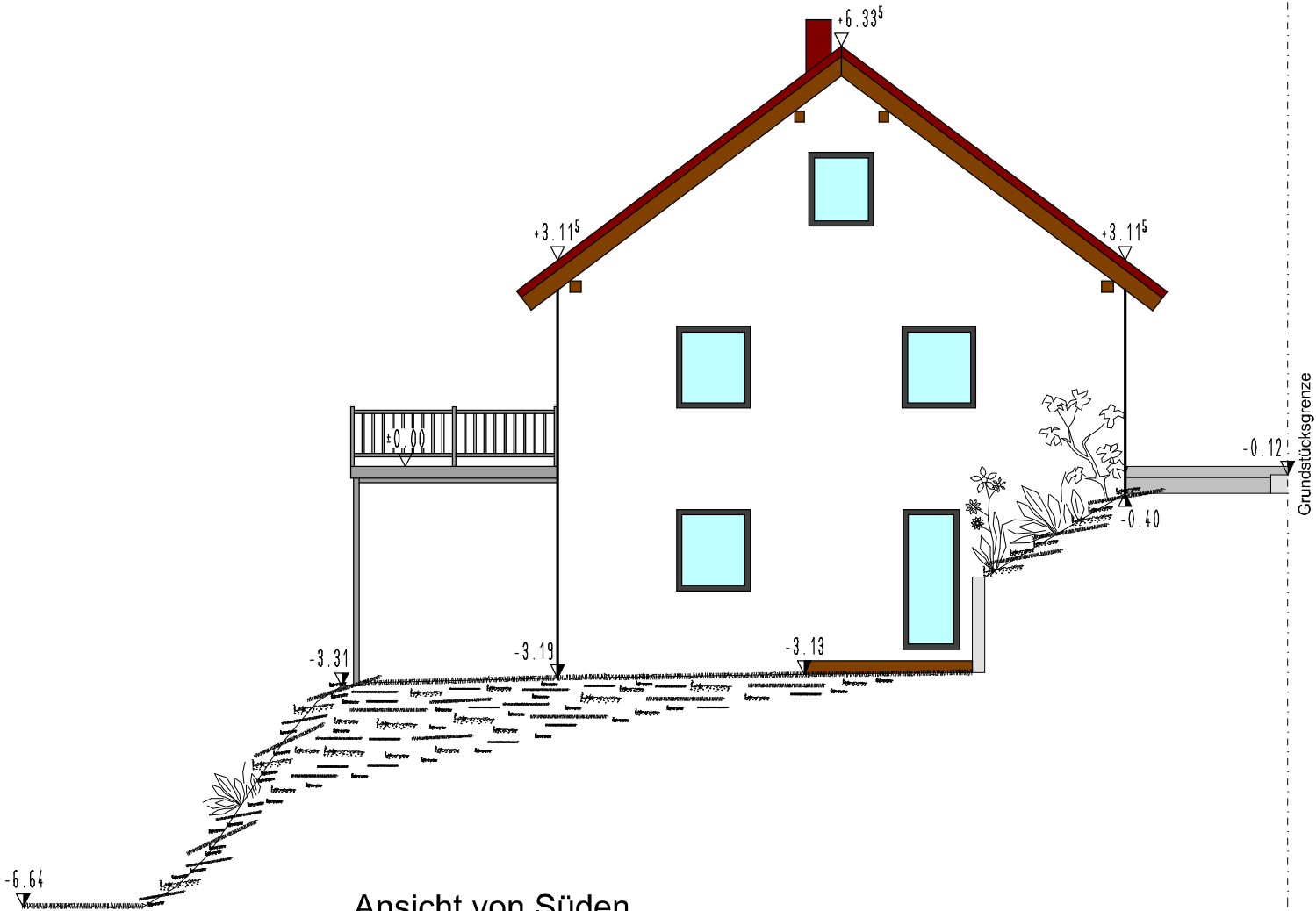
Ansicht von Süden
